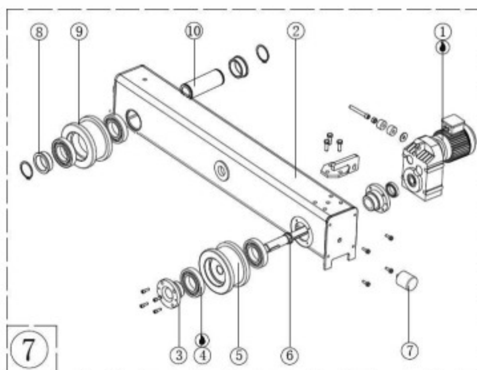
Рисунок 24. Концевая балка
