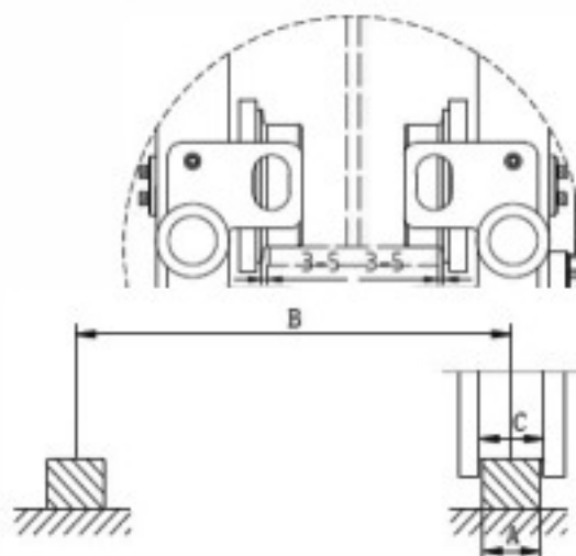
Рисунок 25. Установка крановой тележки
