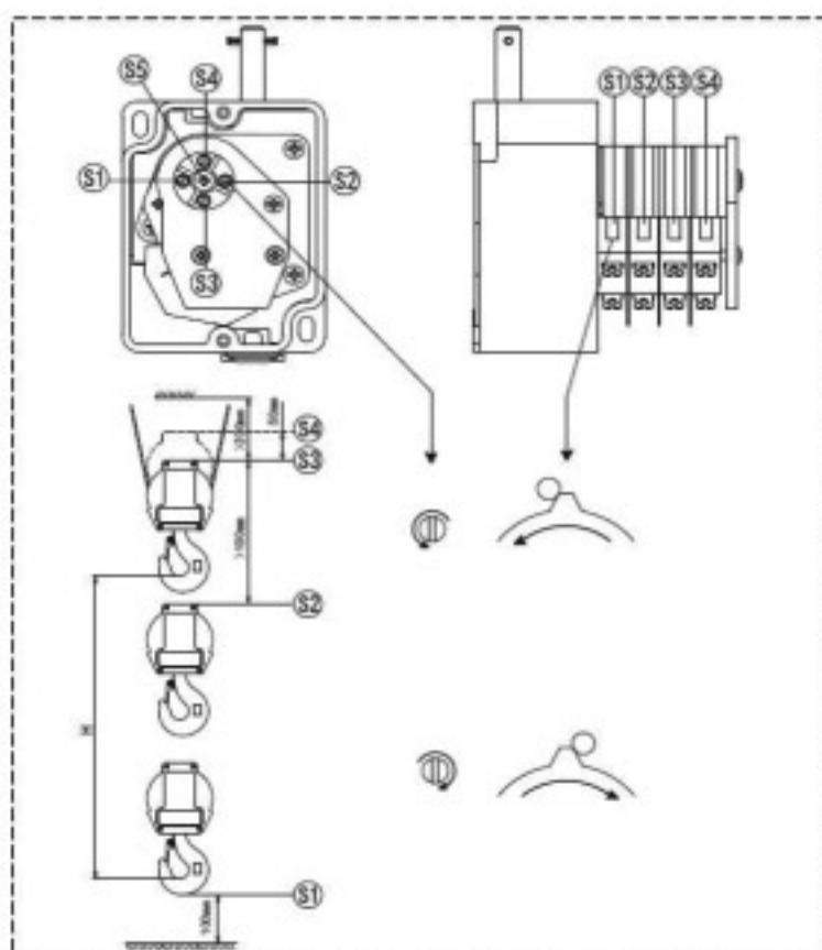
Рисунок 12. Концевой выключатель
