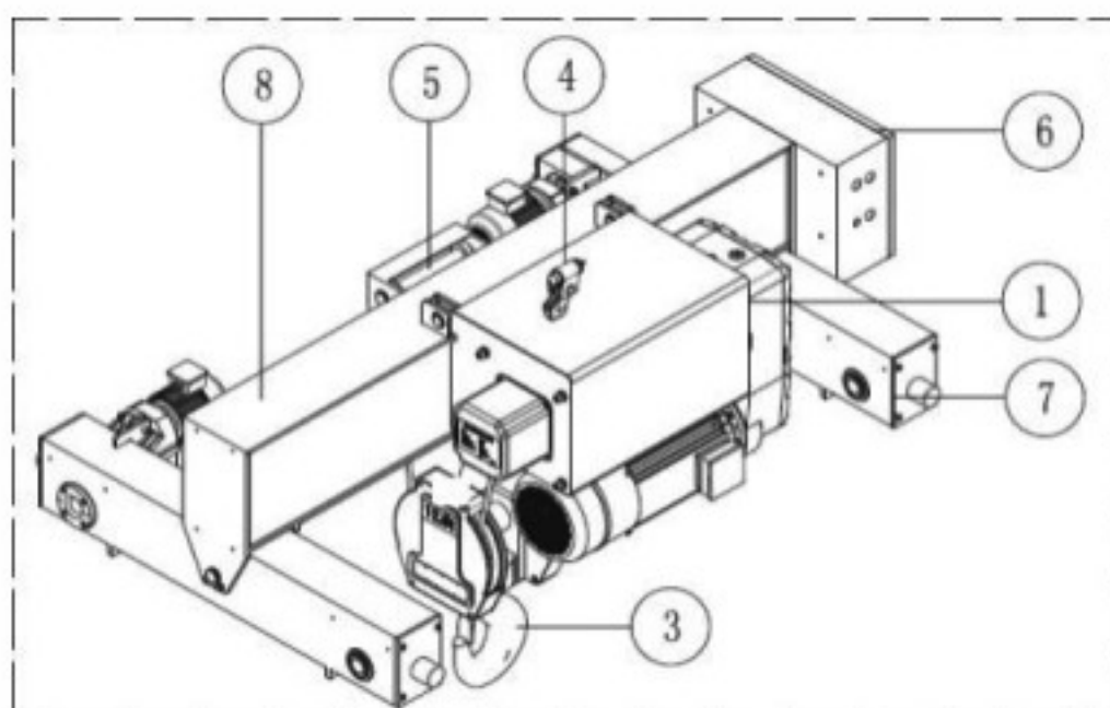
Рисунок 6. Крановая тележка
