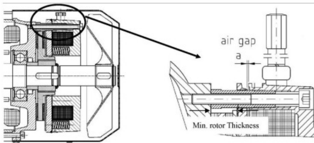
Рисунок 9. Электромагнитный дисковый тормоз
