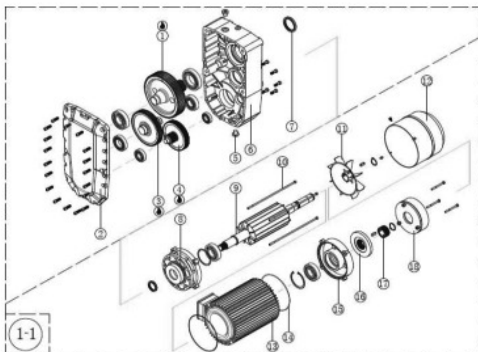
Рисунок 11. Мотор-редуктор подъема
