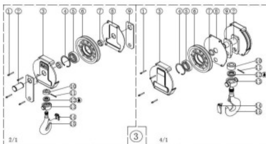
Рисунок 19. Крюковая подвеска
