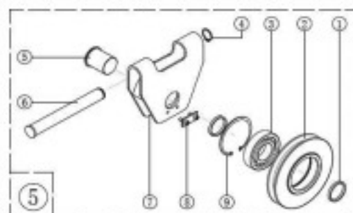
Рисунок 22. Уравнительный блок
