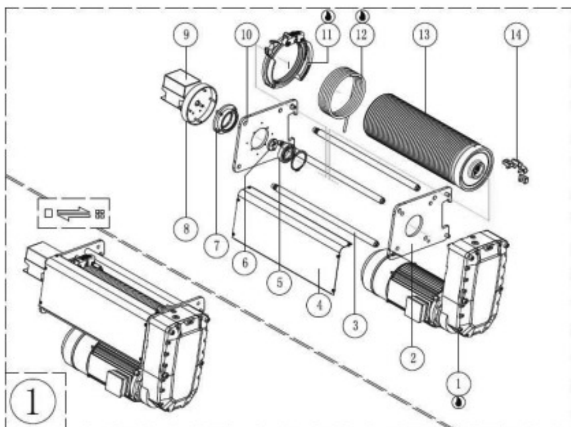
Рисунок 7. Подъемный узел
