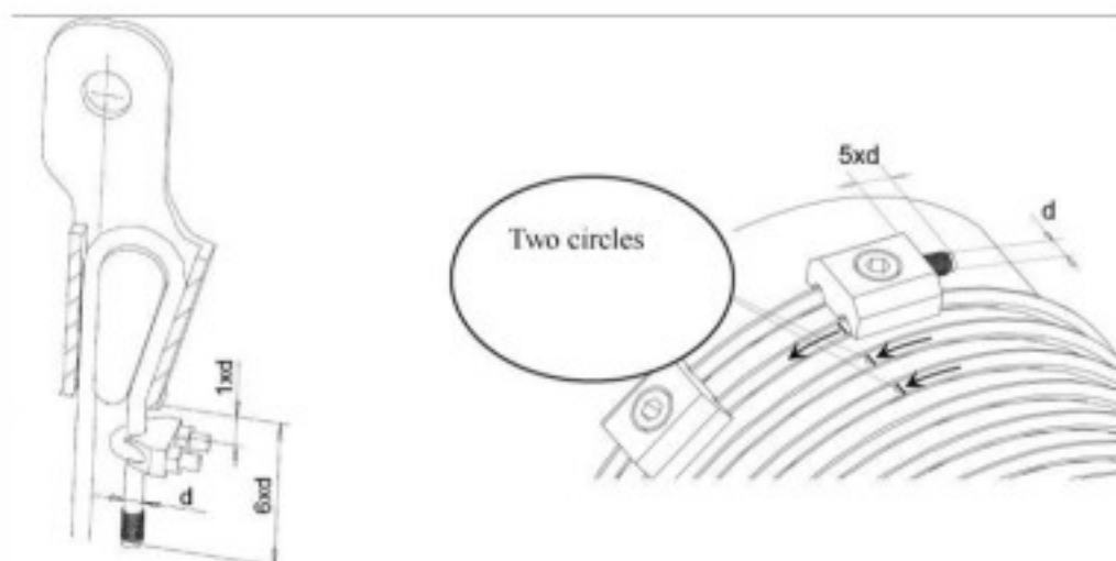
Рисунок 16. Одинарная намотка троса на барабан
