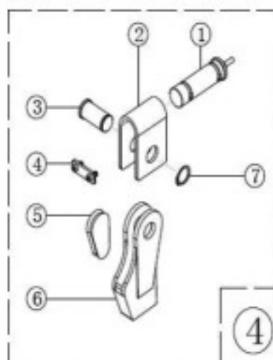
Рисунок 20. Запасовочный узел
