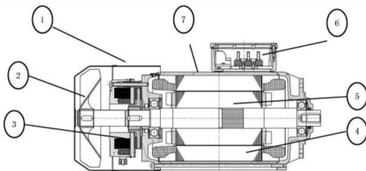
Рисунок 8. Мотор-редуктор подъема
