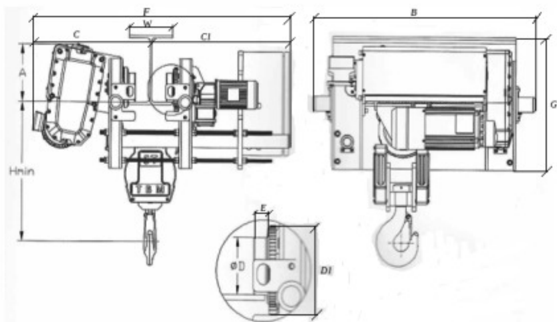
Рисунок 2. Основные параметры тали
