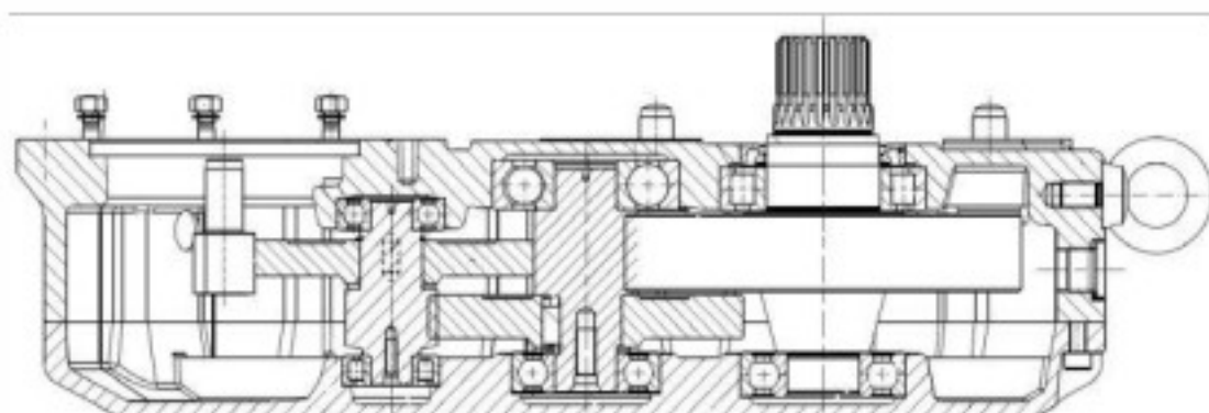
Рисунок 10. Редуктор подъема
