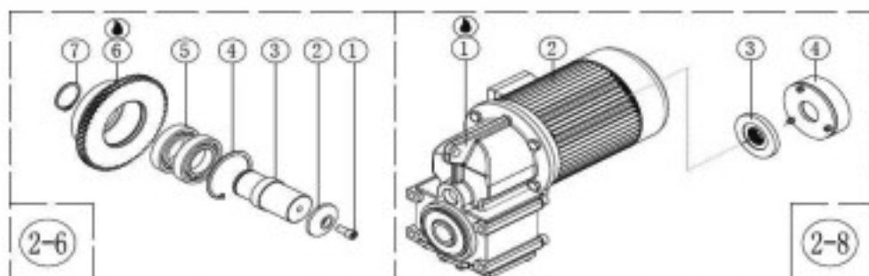
Рисунок 18. Мотор-редуктор передвижения
