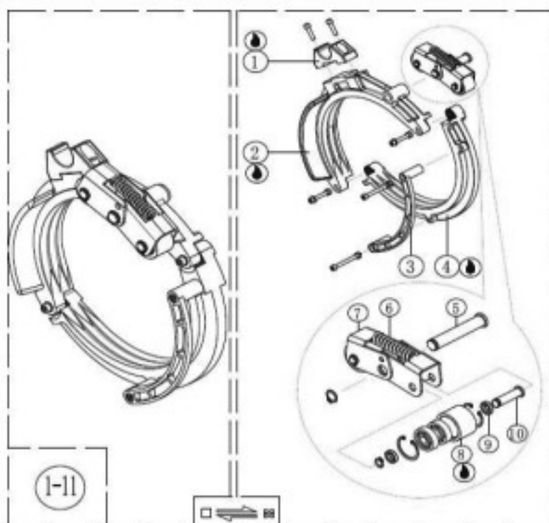
Рисунок 13. Канатоукладчик
