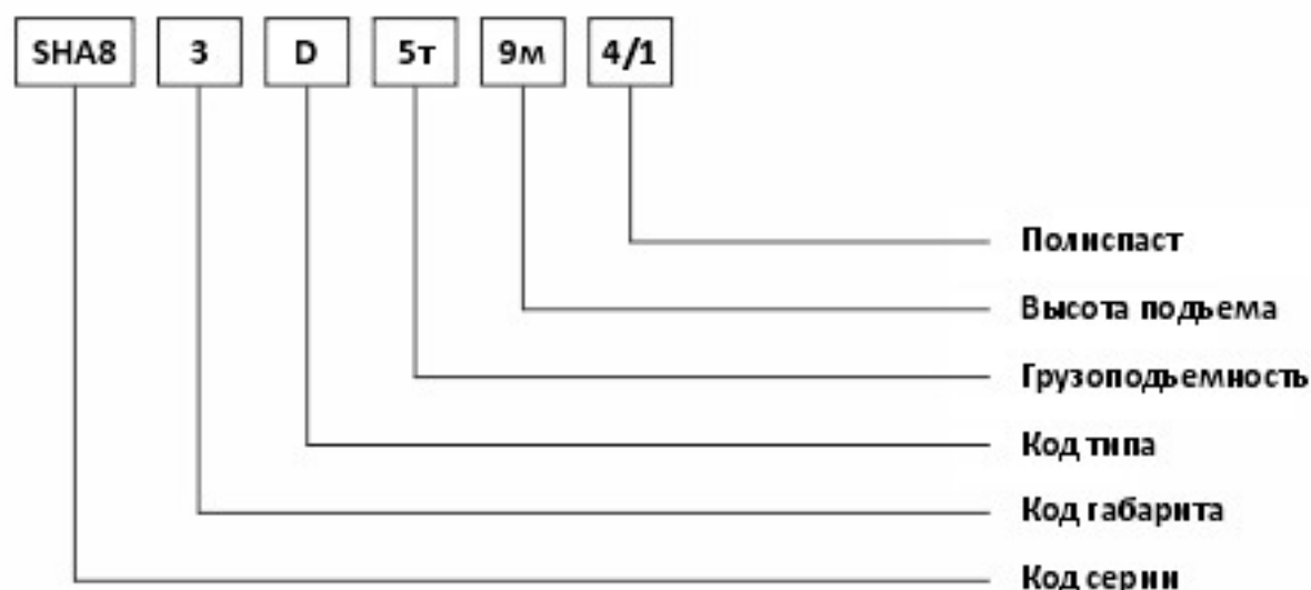
Рисунок 1. Расшифровка маркировки тали
