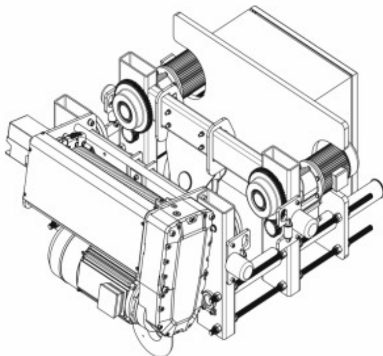
Рисунок 3. Крановая тележка (модификация по специальному заказу)
