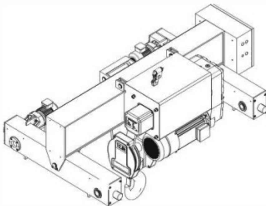
Рисунок 4. Таль подвесного типа UCB
