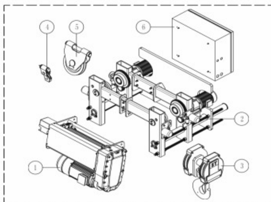
Рисунок 5. Монорельсовая таль с уменьшенной строительной высотой
